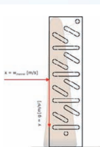
Standardní výměník tepla
