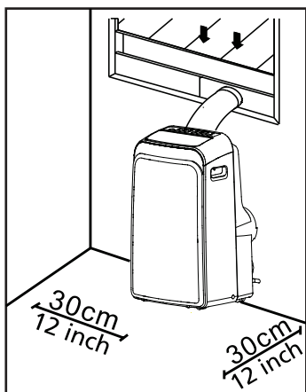
Doporučená instalace
