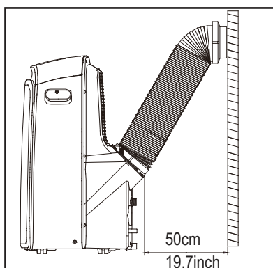
Doporučená instalace
